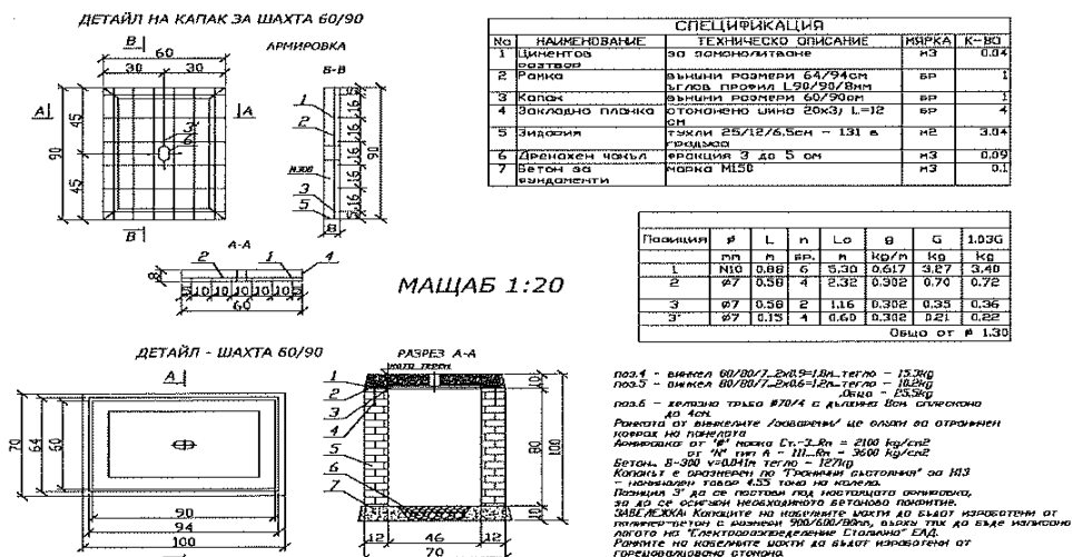
Фиг. 1. Кабелна шахта – единична
